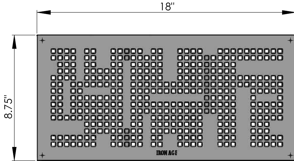
TOP scale 1:4
